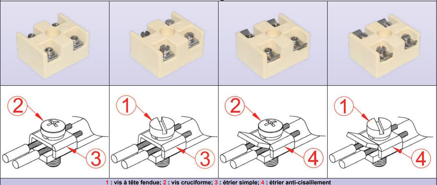
1 : vis à tête fendue; 2 : vis cruciforme; 3 : étrier simple; 4 : étrier anti-cisaillement
